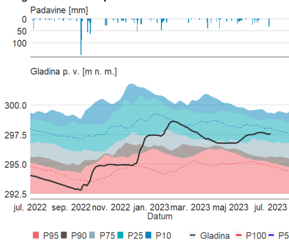
Slika 5. Srednje dnevne gladine podzemnih voda (m.n.v.) v preteklem letu v primerjavi z značilnimi percentilnimi vrednostmi gladin primerjalnega obdobja 1991–2020, zglajenimi s 7 dnevnu drsečim povprečjem in dnevno vsoto padavin območja vodonosnika
