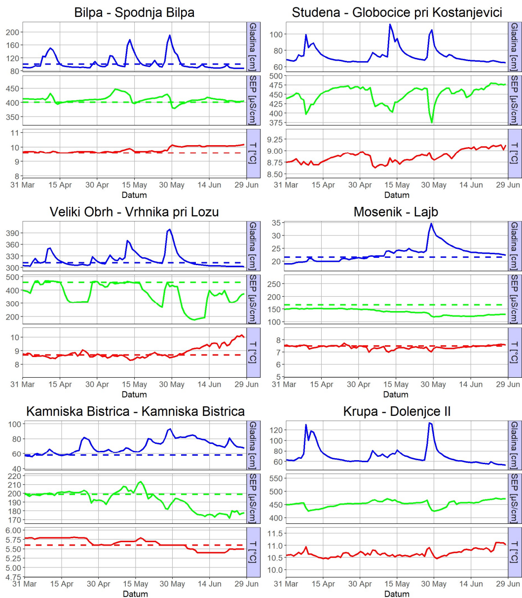
Slika 3. Nihanje vodne gladine (modro), temperature (rdeče) in specifične električne prevodnosti (zeleno) na izbranih merilnih mestih kraških izvirov med aprilom in junijem 2019
