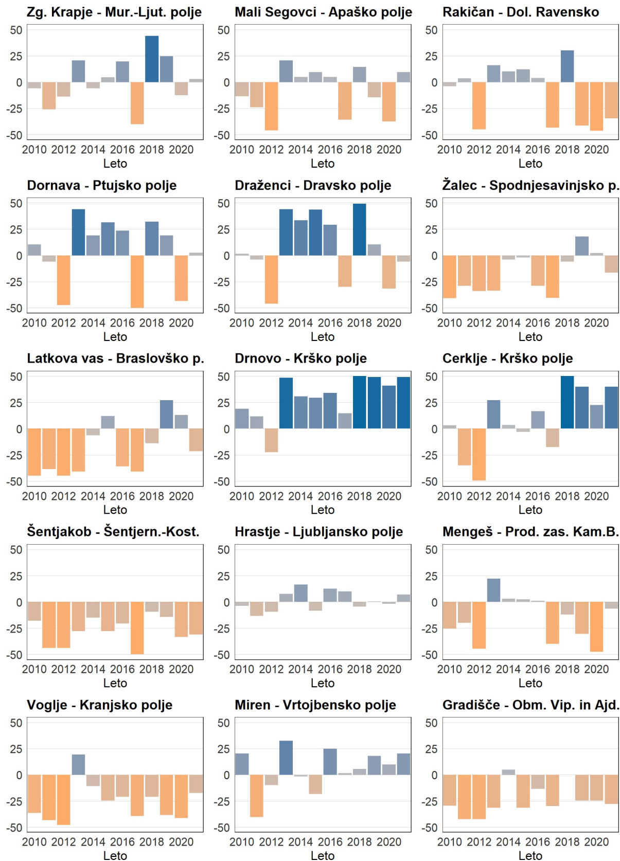
Slika 4. Odklon povprečne julijskih gladine podzemne vode od mediane dolgoletnih julijskih gladin v obdobju 1981–2010, izražene v percentilnih vrednostih Figure 4. Deviation of average July groundwater level in relation from median of long term July groundwater level in period 1981–2010, expressed in percentile values
