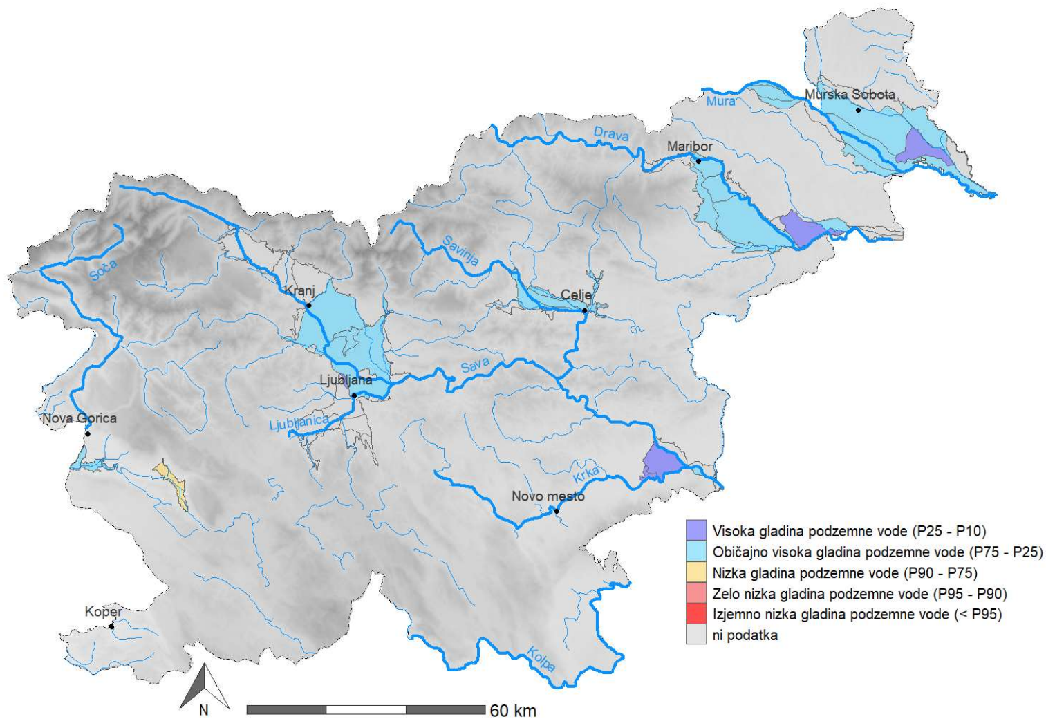
Slika 6. Uvrstitev povprečnih mesečnih gladin podzemne vode v medzrnskih vodonosnikih v percentilne razrede gladin (P) referenčnega obdobja 1991–2020; marec 2023 Figure 6. Average monthly groundwater level in alluvial aquifer classified in percentile values (P) of reference period 1991–2020; March 2022
