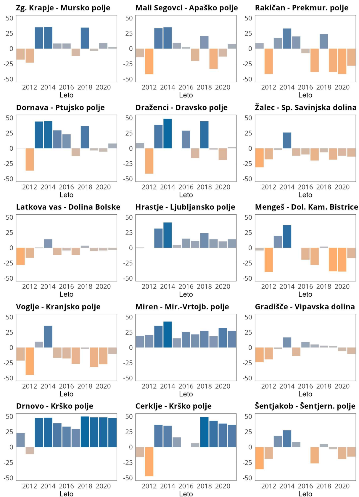
Slika 6. Odklon povprečne gladine podzemne vode v obdobju 2011 - 2021 od mediane dolgoletnih gladin v obdobju 1981 - 2010 izražene v percentilnih vrednostih Figure 6. Deviation of average groundwater level in period from 2011 to 2021 in relation from median of longterm groundwater level in period 1981 – 2010 expressed in percentile values
