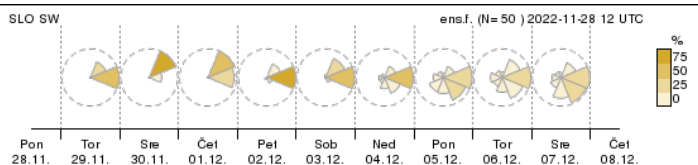
Dnevna porazdelitev smeri vetra na 10m
