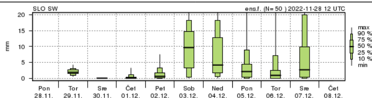
Dnevne skupne padavine
