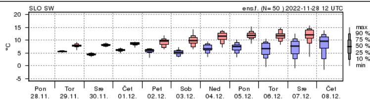
Najnižje in najvišje temperature na 2m
