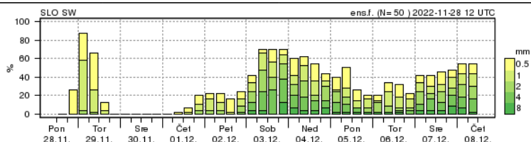
Verjetnost za padavine nad posameznim pragom - v obdobjih po 6 h
