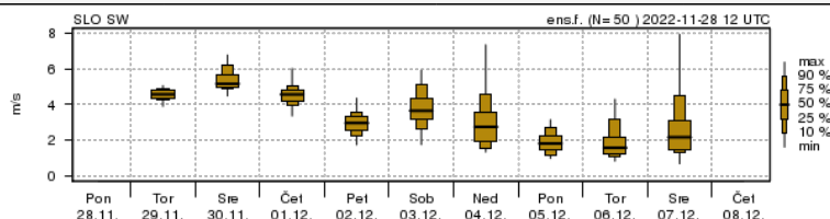
Dnevno povprečje hitrosti vetra na 10m
